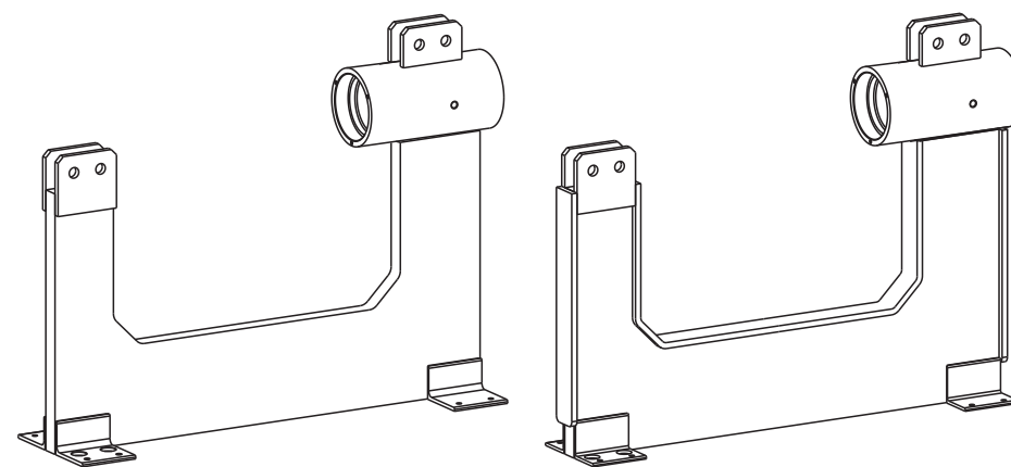
Рис. 2. Отличие усиленной струбцины (справа) от обычной.
